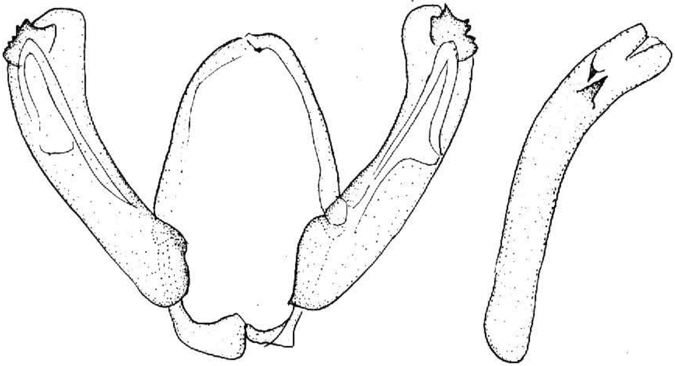
图 526 阴委夜蛾 Athetis funesta (Staudinger) ♂ 外生殖器
